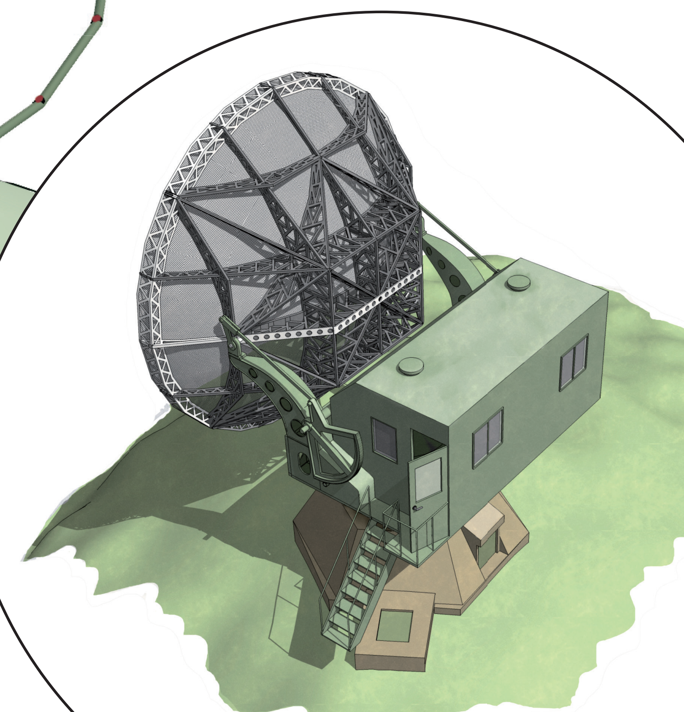
RADAR TYPU "WÜRZBURG-RIESE" "Würzburg-Riese" type radar / "Würzburg-Riese" Funkmessgerät
